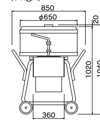
幅850×高さ1040×奥行750
